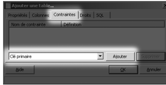
FIGURE 36.16 – Ajout d'une contrainte de clé primaire
