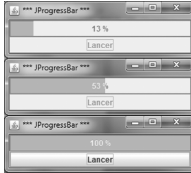
FIGURE 29.15 – Une JProgressBar
