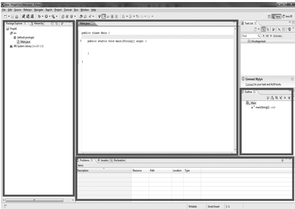
FIGURE 1.15 – Fenêtre principale
