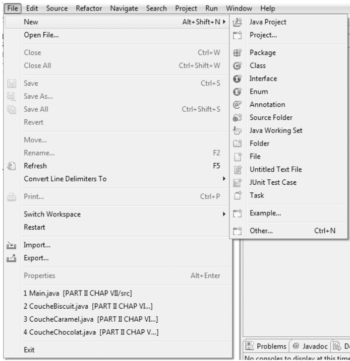
FIGURE 1.7 – Menu « File »
