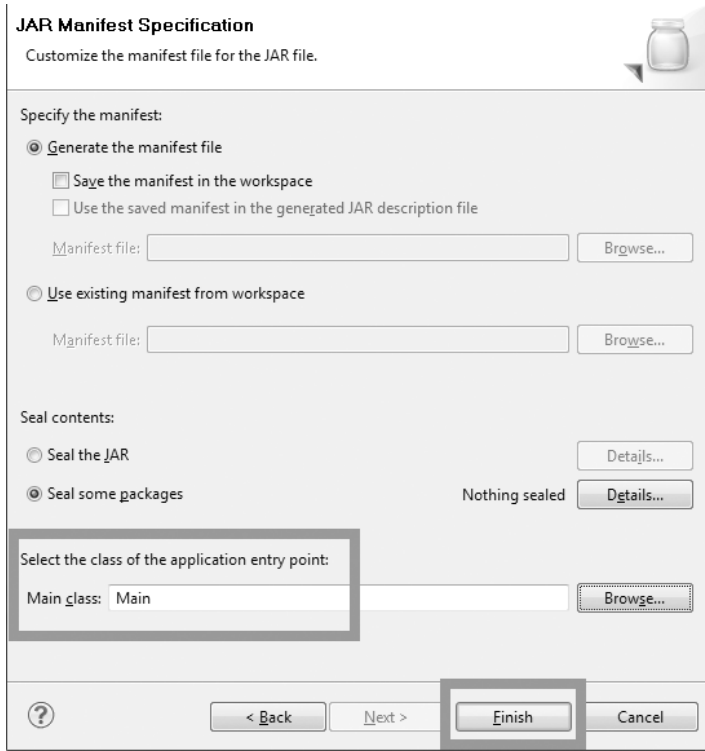
FIGURE 24.8 – Récapitulatif d'export
