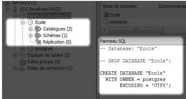
FIGURE 36.11 – Première BDD
