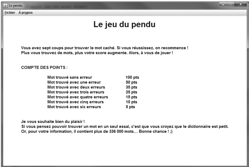
FIGURE 32.1 – Écran principal
