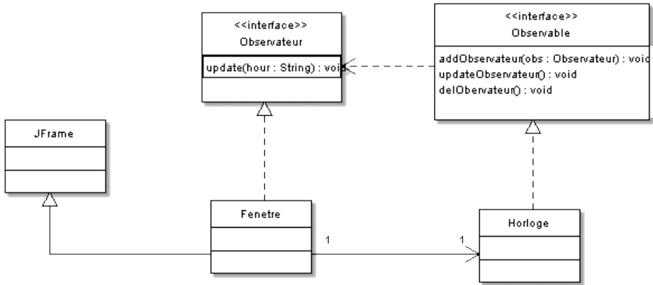
FIGURE 23.18 – Diagramme de classes du pattern observer
